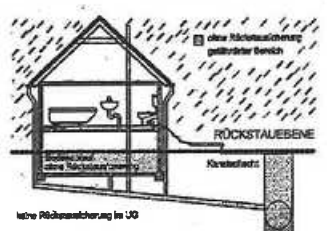
Bild 1: Kanalarückstau ohne Rückstausicherungen
