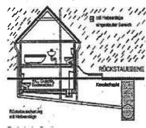
Bild 3: Kanalarückstau bei Einbau einer Hebeanlage als Rückstausicherungen
