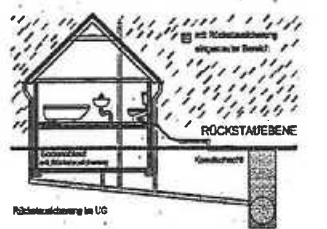
Bild 2: Kanalarückstau mit Rückstausicherungen
