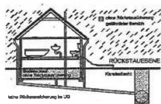
Bild 1: Kanalrückstau ohne Rückstausicherungen
